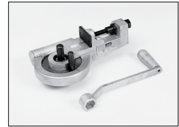
Fig. R8 — 412 Bender
