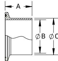
BPE Table DT-4.1.4-1 ASME BPE 2019
