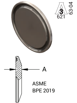
BPE Table DT-4.1.5-2
