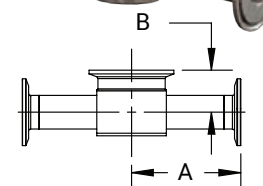
BPE Table DT-4.1.2-11 ASME BPE 2019
