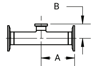
BPE Table DT-4.1.2-9 ASME BPE 2019
