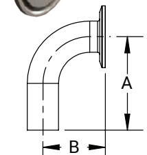
BPE Table DT-4.1.1-2 ASME BPE 2019
