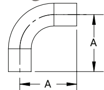
BPE Table DT-4.1.1-1 ASME BPE 2019
