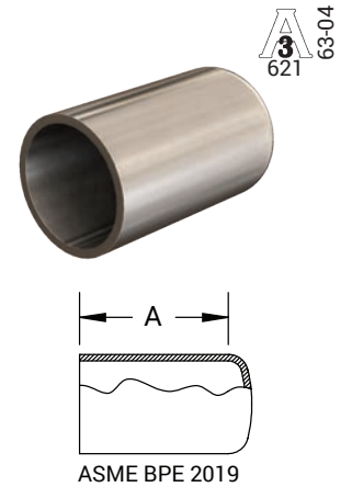
BPE Table DT-4.1.5-1
