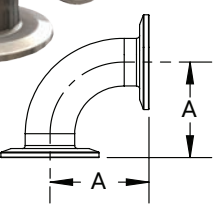
BPE Table DT-4.1.1-3 ASME BPE 2019
